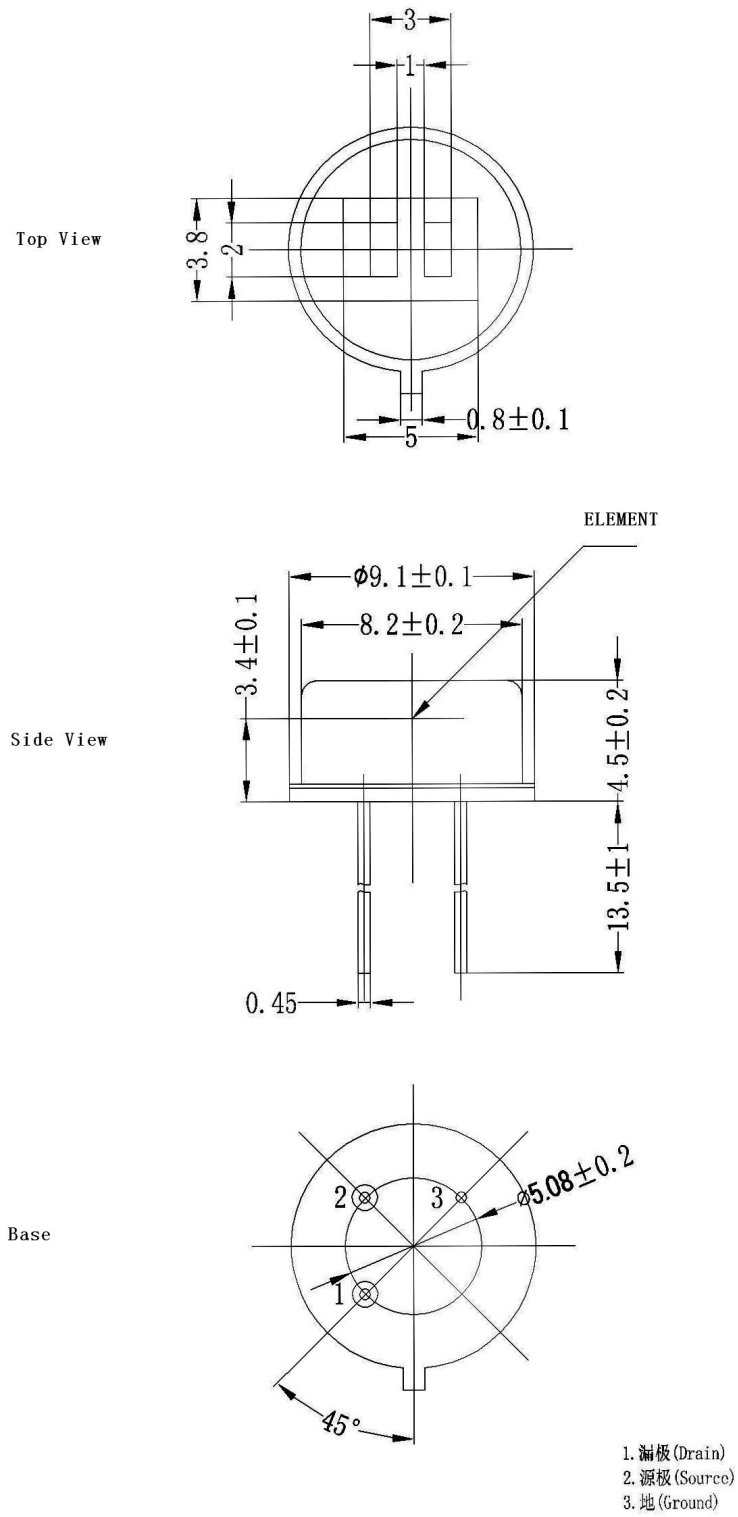
图 1 尺寸规格图
